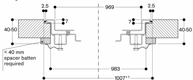
Longitudinal section
