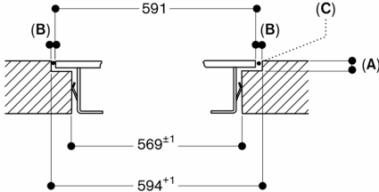
Longitudinal section
