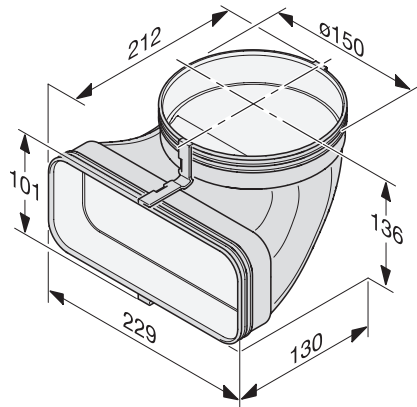
DFK-AK90, Adapter kurz, eckig-rund 90°, Skizze
