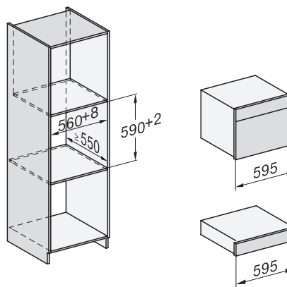
Einbau_DG_DGM_DGC_XL_ESW7x10_EVS7010 Skizze
