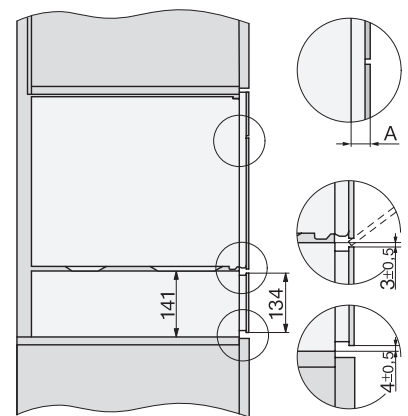
Seitenansicht_DG_DGM_ESW7x10_EVS7010, Skizze
