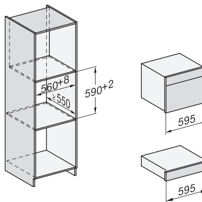
Einbau_DG_DGM_DGC_XL_ESW7x10_EVS7010 Skizze
