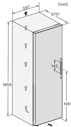
FNS4882D, Aufstellskizze
