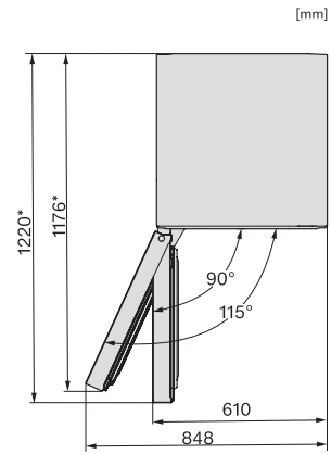
FNS4882D, Draufsicht
