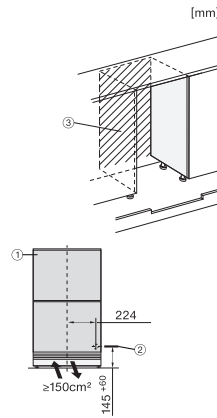
KU7175D, Built-under, Installationskizze (*Fußnote)
